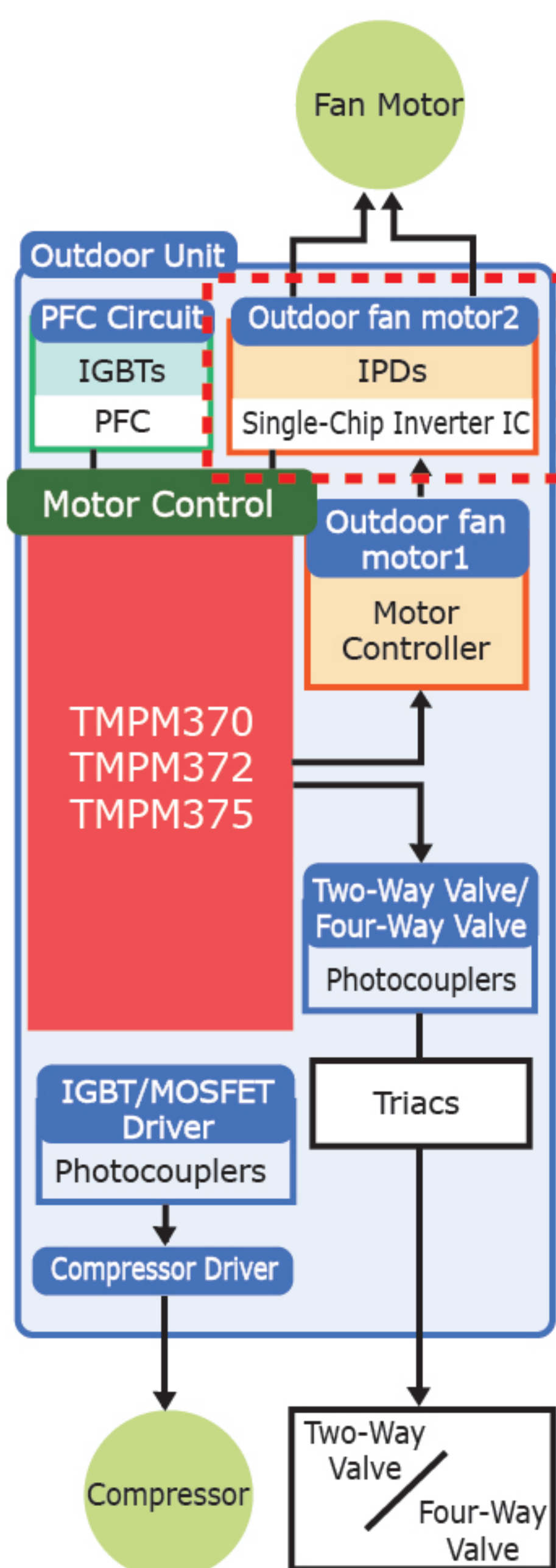
系统框图
