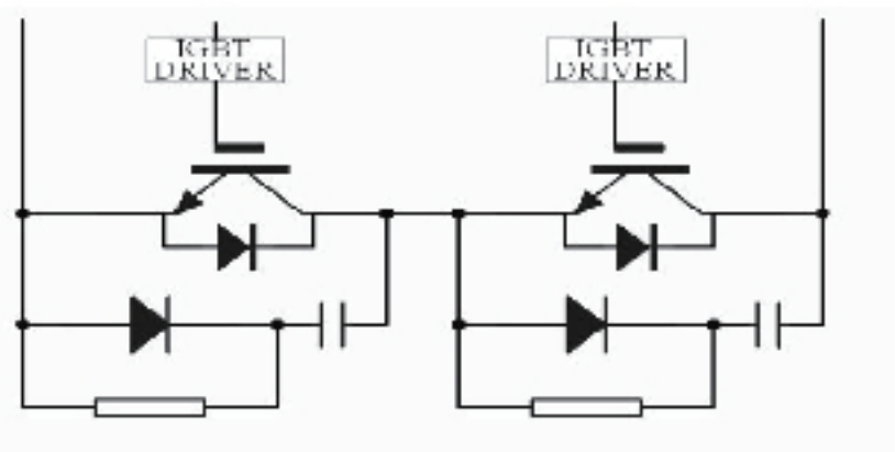
二电平拓扑
