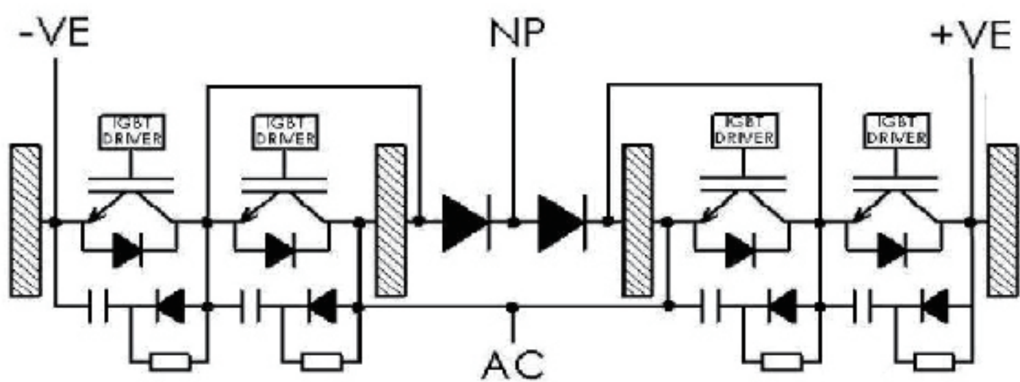
三电平拓扑
