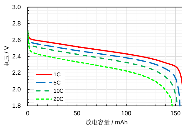
放电特性
