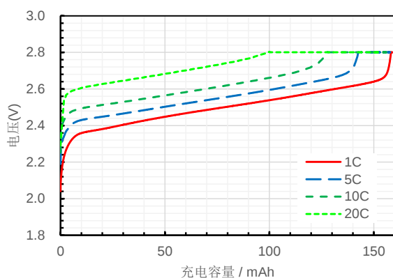
充电特性
