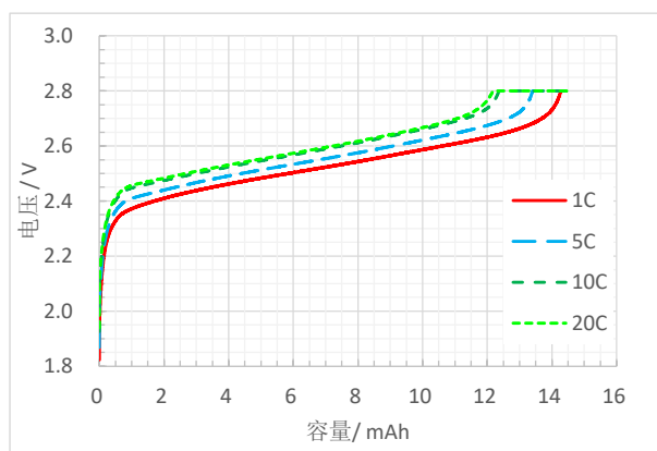
充电特性
