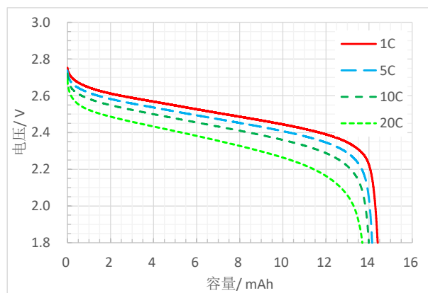
放电特性
