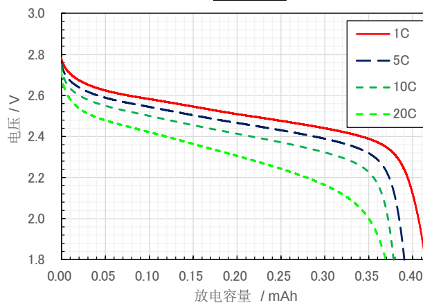
放电特性
