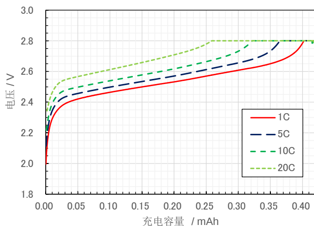
充电特性
