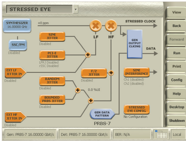
压力眼图视图
