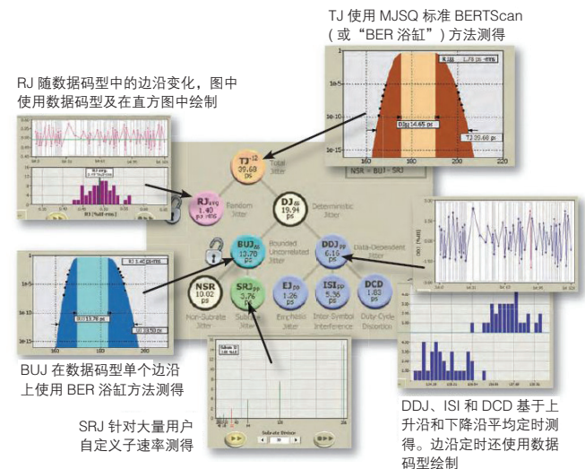
抖动分离及定位。
