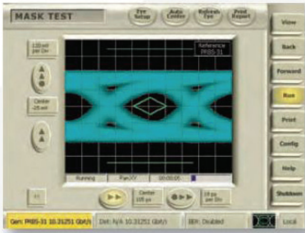
XFI 电特性压力眼图一致性测试
