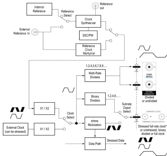
BSX 系列带压力测试能力模块的时钟路径功能方框图
