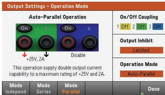
图 4. 自动并联操作使输出电流增加一倍。
