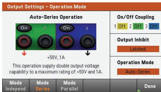
图 3. 自动串联操作使输出电压增加一倍。
